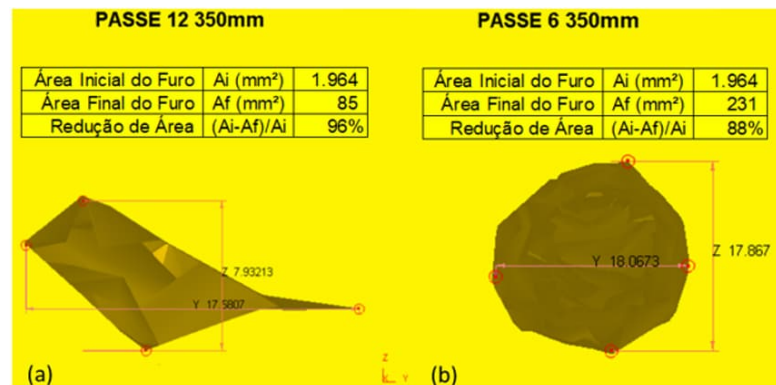
Figura 61 – Dimensão do vazio (furo) “passo Oit 350 mm”: (a) 2 bigornas, redução de área do vazio igual a 96%; (b) 4DFD, redução de área do vazio igual a 88%.
