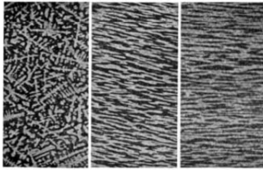
Figura 15 – Efeito do trabalho a quente na estrutura do lingote. [10]
