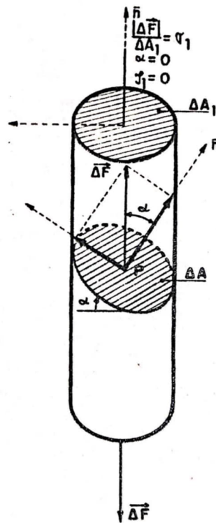
Figura 2 – Tensões em diferentes planos de corte na tração de um cilindro, com uniforme distribuição de forças em qualquer seção do corpo, tais como \Delta A e \Delta A_1 . [1]
