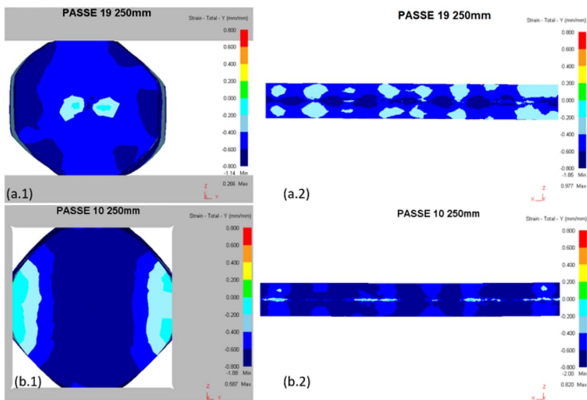
Figura 78 – Deformação total direcional Y “passe Oit 250 mm”: (a.1) 2 bigornas corte transversal e (a.2) corte longitudinal; (b.1) 4DFD corte transversal e (b.2) corte longitudinal; componentes compressivas elevadas para os dois processos, porém maior para o processo 4DFD (cores azul escuro e azul mais predominantes).
