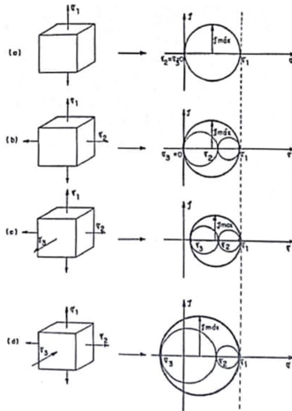
Figura 7 – Exemplos de círculos de Mohr para diferentes estados de tensão. [1]
