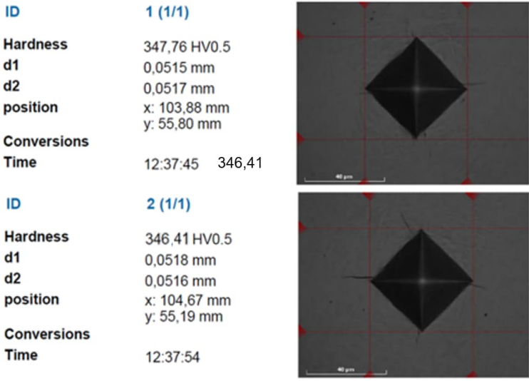
Figura 90 – Microdurezas “Vickers” medidas na carepa compactada da região central da fatia 4D-4 e resultados encontrados iguais a 347,76 HV0.5 (329 HB) e 346,41 HV0.5 (328 HB).
