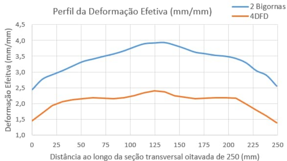
Figura 76 – Perfis das deformações efetivas ao longo da seções transversais no “passe Oit 250 mm” relacionada à Figura 75 (a.1) e (b.1) dos processos 2 bigornas e 4DFD, respectivamente: valores mais baixos nas superfícies (0 e 250 mm) iguais a 2,5 mm/mm (2 bigornas) e 1,4 mm/mm (4DFD); valores mais altos nos centros (125 mm) iguais a 3,9 mm/mm (2 bigornas) e 2,4 mm/mm (4DFD).
