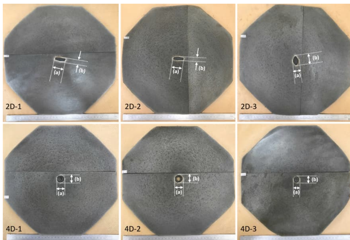
Figura 85 – Macrografias das fatias no formato oitavado 350 mm: 2 bigornas planas (2D-1, 2D-2 e 2D-3); dispositivo 4DFD (4D-1, 4D-2 e 4D-3); dimensões (a) e (b) dos vazios encontram-se na Tabela 12.
