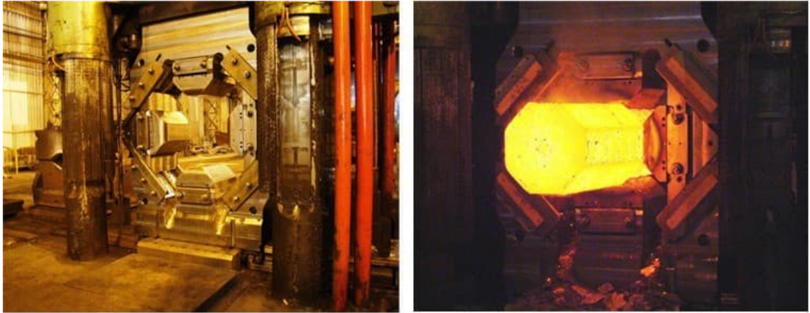
Figura 45 – Fotografias do dispositivo 4DFD montado na prensa P.3000T (esquerda) e durante um forjamento (direita).
