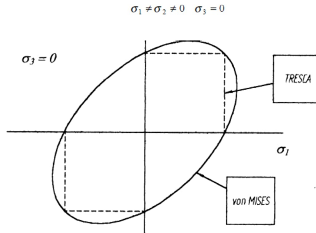
Figura 11 – Comparação entre os critérios de TRESCA e von MISES. [2, 37]
