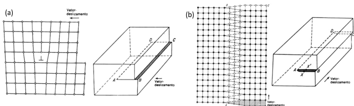
Figura 9 – Representações das discordâncias: (a) em cunha; (b) em hélice. [2, 37]
