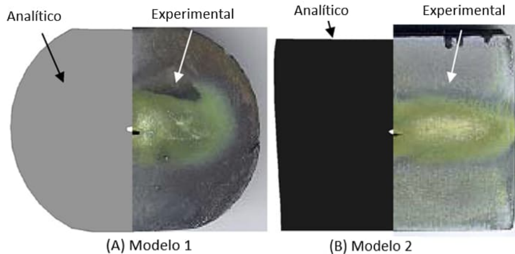
Figura 31 – Comparação da forma da seção transversal com o resultado experimental (direita) e o resultado analítico (esquerda). Adaptado de [23].
