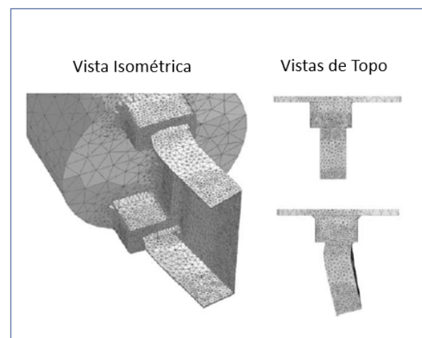
Figura 37 – Esquema representativo da simulação de um processo de extrusão do fluxo do material, mostra a curvatura em vistas isométrica e de topo. Adaptado de [28].
