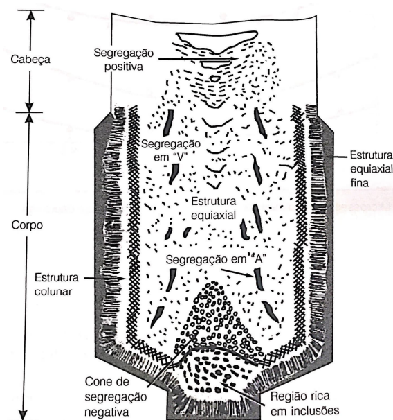
Figura 14 – Estrutura primária de um lingote do processo de lingotamento convencional. [8]
