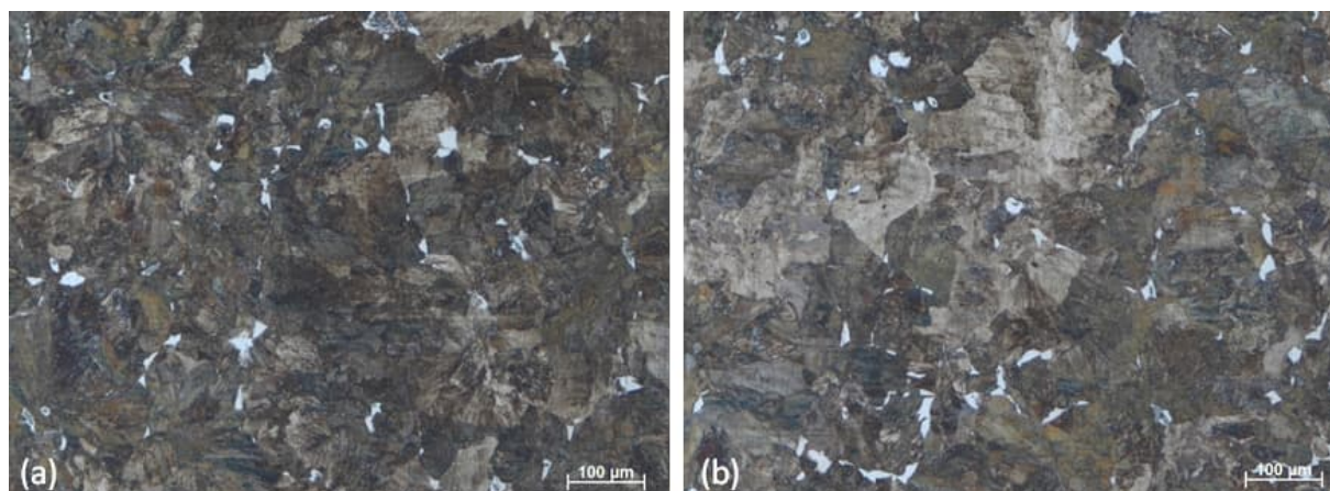
Figura 96 – Micrografias do núcleo do oitavado 250 mm: (a) 2 bigornas; (b) 4DFD; microestrutura perlítica e ferrítica; granulação igual a 3 ASTM para os dois processos. Ataque Nital 4%. Aumento 100x.
