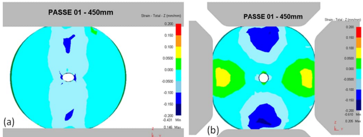
Figura 58 – Deformação total direcional Z no “passe 1”: (a) 2 bigornas, as resultantes das deformações, que eram trativas na direção Y da Figura 57, passam a ser somente compressivas (cores azul turquesa e azul) em torno do vazio na direção Z; (b) 4DFD, maior presença das deformações negativas (cor azul turquesa) em torno do vazio, mas, as pequenas resultantes das deformações positivas (cor verde) mudam de sentido para direção Z quando comparadas às resultantes da direção Y da Figura 57.
