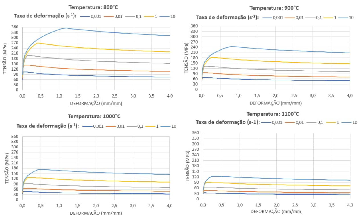
Figura 43 – Curvas de tensão-deformação do aço AISI 4145, com os fluxos de escoamentos calculados com o software JMatPro® [31], para as temperaturas de 800°C, 900°C, 1000°C e 1100°C. As taxas de deformação do presente trabalho foram entre 0,188 e 0,375 s -1 , conforme apresentado na Tabela 7.
