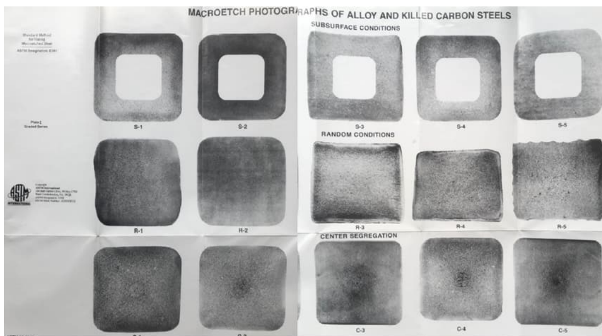
Figura 50 – “Quadro I” da especificação ASTM E381– 20 com série graduada da segregação de três condições: sub superfície (S); meio raio (R); centro (C). [33]
