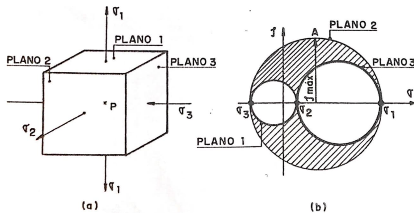
Figura 6 – Extensão do círculo de Mohr a três dimensões. [1]
