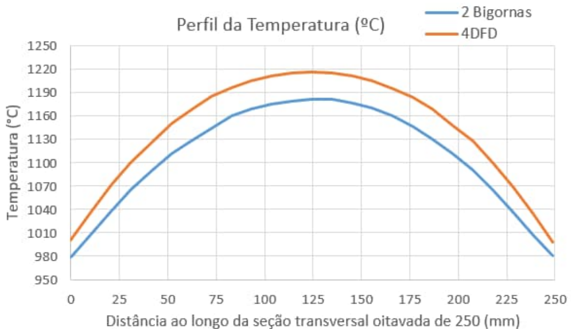
Figura 71 – Perfil térmico ao longo da seção transversal no “passe Oit 250 mm”: temperaturas mais baixas nas superfícies (0 e 250 mm) iguais a 979°C (2 bigornas) e 999°C (4DFD); temperaturas mais altas nos centros das barras (125 mm) iguais a 1181°C (2 bigornas) e 1217°C (4DFD).
