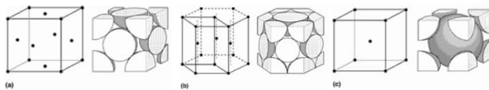
Figura 8 - Principais estruturas cristalinas dos metais: (a) CFC; (b) HC; (c) CCC. [3]
