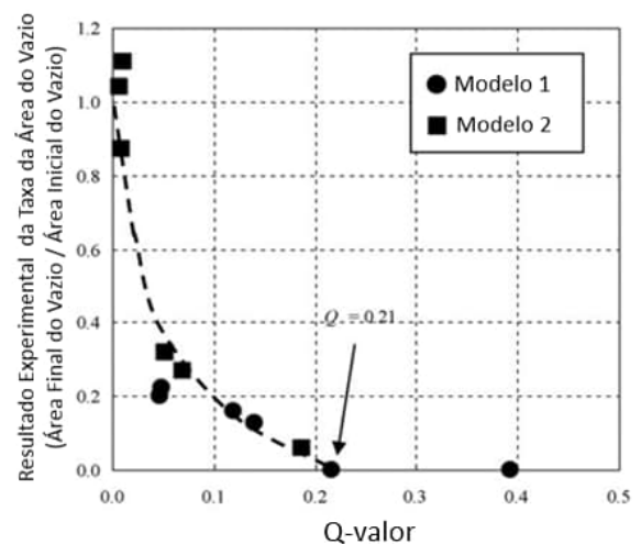
Figura 33 – Valor Q analítico versus a taxa da área do vazio experimental. Adaptado de [23].
