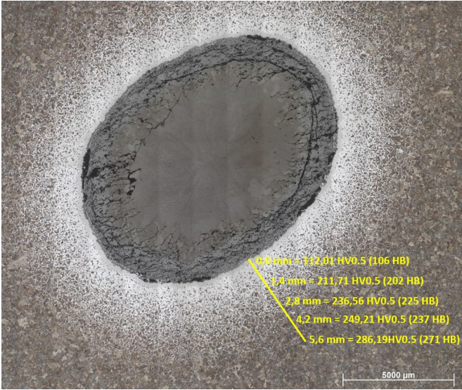
Figura 91 – Micrografia do mosaico do vazio na região central da fatia 4D-4 com os resultados das microdurezas “Vickers” (convertidas em “Brinell”) medidas no aço base. Ataque Nital 4%. Aumento 5x.
