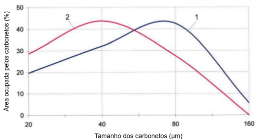
Figura 20 – Distribuição de carbonetos: forjamento rotativo radial “1” e “4DFD”. Adaptado de [12].
