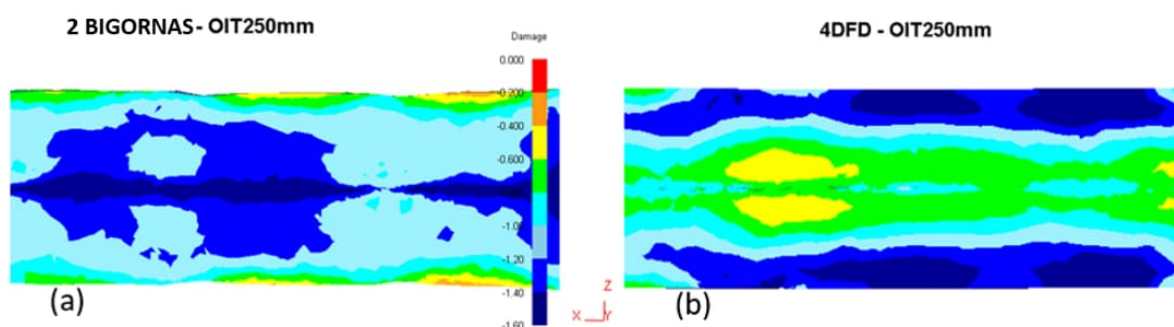
Figura 81 – Parâmetro Q -valor no “passe Oit 250 mm”: (a) 2 bigornas, valor igual a 1,4 \pm 0,2 (cores azul e azul escuro); (b) 4DFD, valor igual a 0,8 \pm 0,2 (cores verde e azul turquesa).
