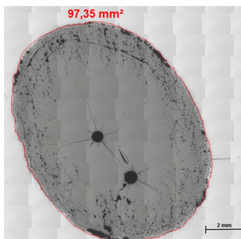
Figura 88 – Mosaico com a área do vazio igual a 97,35 mm 2 (fatia 4D-4). As duas impressões redondas de durezas “Rockwell” na carepa compactada foram desconsideradas porque o melhor processo de medição nesta condição é a microdureza “Vickers”. Aumento 5x.
