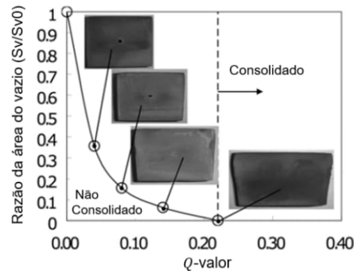
Figura 25 – Variação da razão da área do vazio ( S_v/S_{v0} , área final dividida pela área inicial do vazio) com o Q -valor, equação (41). Adaptado de [22].
