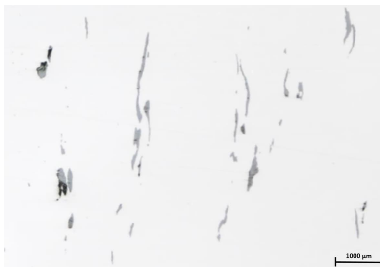
Figura 87 – Micrografia da região segregada retirada da fatia 2D-4 da região do meio raio no sentido longitudinal da barra forjada no oitavado de 250 mm; presença de sulfetos de manganês, desejados na estrutura deste aço para facilitar processos de usinagem. Sem ataque. Aumento 100x.
