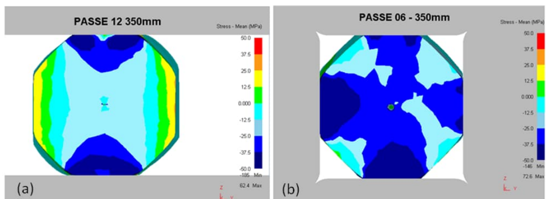
Figura 62 – Tensão hidrostática no “passo Oit 350 mm”: (a) 2 bigornas, tensões de compressão intermediárias (cores azul e azul claro); (b) 4DFD, tensões de compressão mais elevadas (cores azul e azul escuro).
