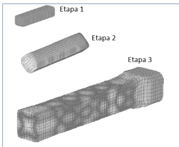
Figura 36 – Esquema representativo da simulação dos contornos da temperatura em três etapas da deformação de um processo de forjamento por estiramento. Adaptado de [28].
