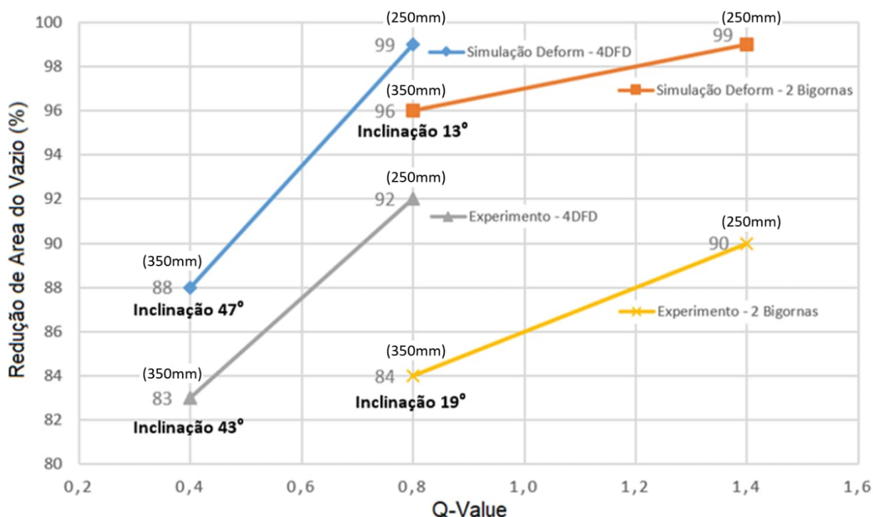
Figura 92 – Redução de área do vazio e Q -valor, após simulações no DEFORM™-3D [26] (Simulação Deform - 2 Bigornas e Simulação Deform - 4DFD) e execuções dos experimentos com o forjamento na prensa P3.000T (Experimento - 2 Bigornas e Experimento - 4DFD). Há coerência entre os modelos numérico e experimental: quanto maior o Q -valor, maior é a tendência do fechamento dos vazios com o aumento das suas reduções de área; a tendência do fechamento do vazio foi mantida, o que é comprovado pela proximidade das inclinações das retas de cada processo.
