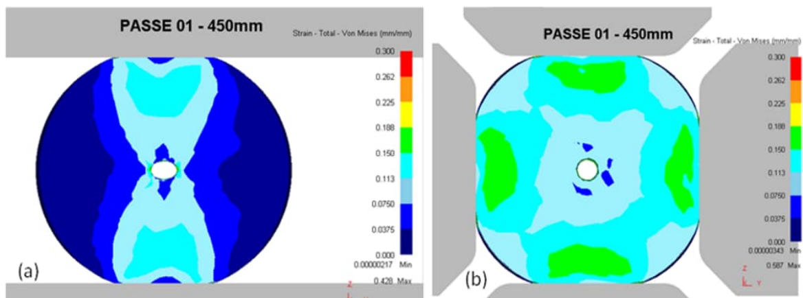
Figura 56 – Deformação de von Mises no “passe 1”: (a) 2 bigornas, a maior deformação efetiva localizou-se somente na faixa central (cores azul turquesa e azul na direção Z); (b) 4DFD, deformação efetiva distribuída ao longo de toda seção transversal (cor azul turquesa no centro e meio raio, além da cor verde próxima das bigornas).
