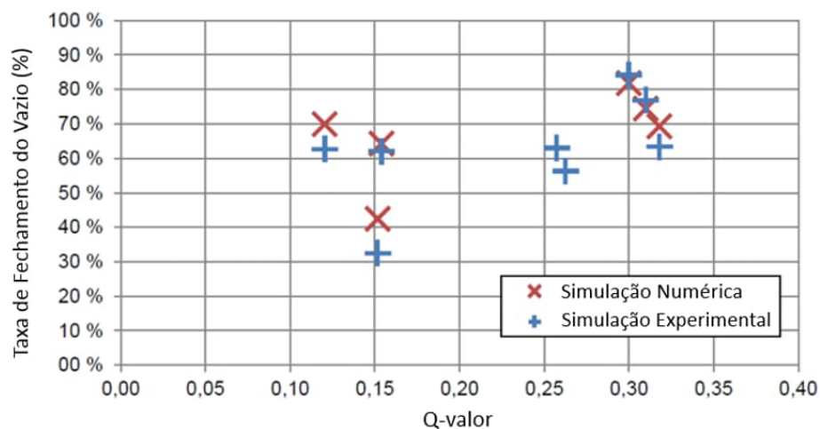
Figura 34 – Taxa de fechamento e Q -valor de simulações experimental e numérica. Adaptado de [9].
