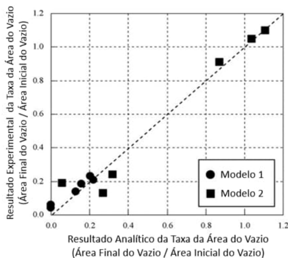
Figura 32 – Taxa da área do vazio do resultado analítico versus experimental. Adaptado de [23].
