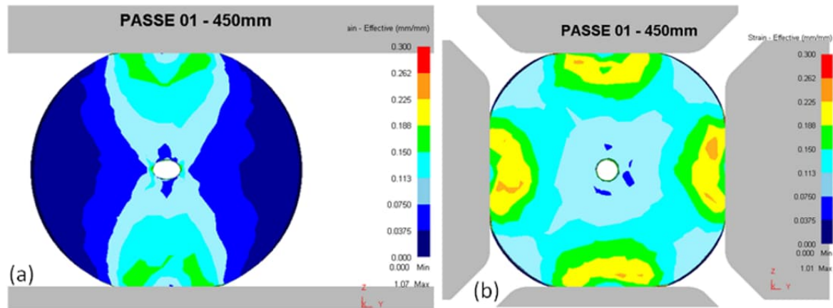
Figura 55 – Deformação efetiva no “passe 1”: (a) 2 bigornas, a maior deformação efetiva localizou-se somente na faixa central (cores azul turquesa e azul na direção Z); (b) 4DFD, deformação efetiva distribuída ao longo de toda seção transversal (cor azul turquesa no centro e meio raio, além da cor verde próxima das bigornas).
