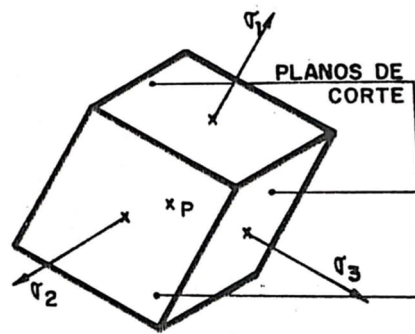
Figura 3 – Planos passando pelo ponto P , onde \tau = 0 . [1]
