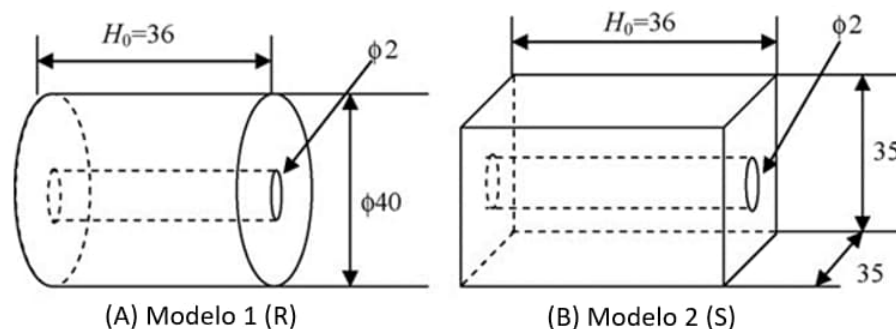
Figura 27 – Formato inicial do material experimental: (A) Modelo 1 (R, redondo); (B) Modelo 2 (S, quadrado); Dimensões em milímetros; H_0 é o comprimento inicial. Adaptado de [23] .
