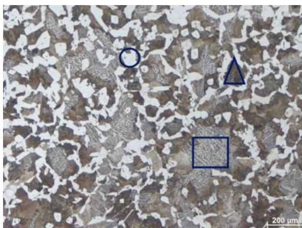
Figura 93 – Micrografia das regiões de microdurezas “Vickers” a 2,8 mm do vazio da Figura 91, ainda na camada descarbonetada, nas fases presentes: região do círculo com a ferrita pró-eutetóide, 145,98 HV0,5 (140 HB); região do quadrado com a perlita grosseira, 281,47 HV0,5 (267 HB); e região do triângulo com a perlita fina, 314,23 HV0,5 (297 HB). Ataque Nital 4%. Aumento 50x.
