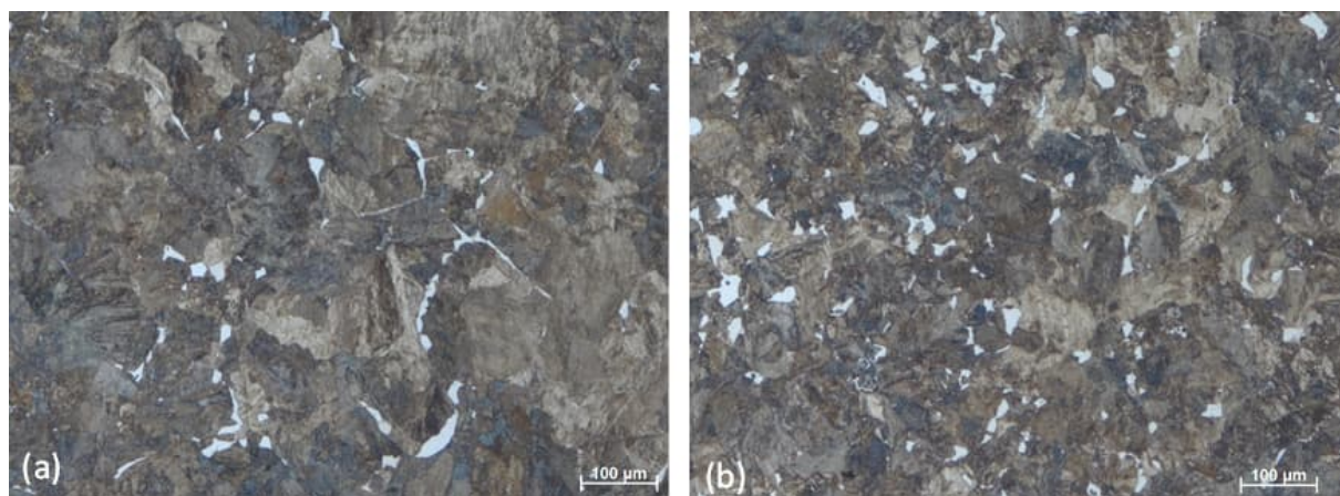
Figura 95 – Micrografias do meio raio do oitavado 250 mm: (a) 2 bigornas; (b) 4DFD; microestrutura perlítica e ferrítica; tamanho de grão mais grosseiro para o processo com 2 bigornas, com 2 ASTM, do que para o 4DFD, igual a 4 ASTM. Ataque Nital 4%. Aumento 100x.
