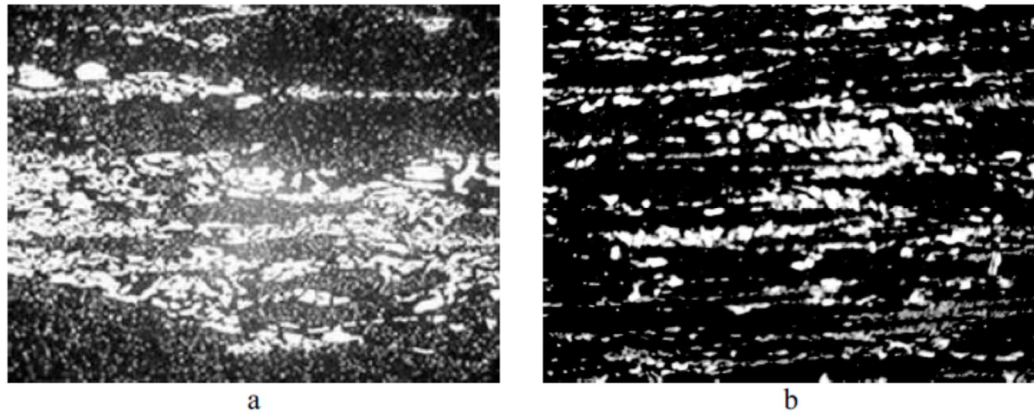
Figura 21 – Micrografia ótica dos carbonetos no núcleo da barra redonda 122 mm: (a) forjamento rotativo radial; (b) 4DFD; aumento 100X. [12]
