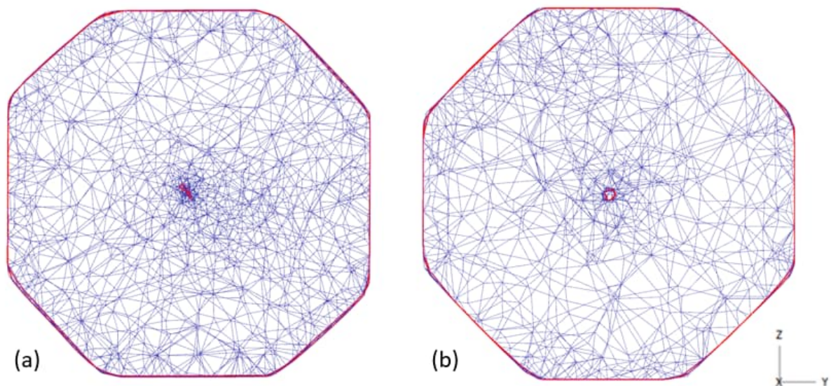
Figura 72 – Remodelagem da malha da furação ao final do último passe: (a) 2 bigornas; (b) 4DFD.
