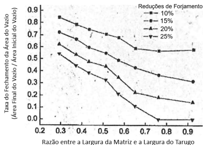
Figura 38 – Taxa do fechamento do vazio em função da razão entre a largura da matriz (ou bigorna) e a largura do tarugo. Adaptado de [29].
