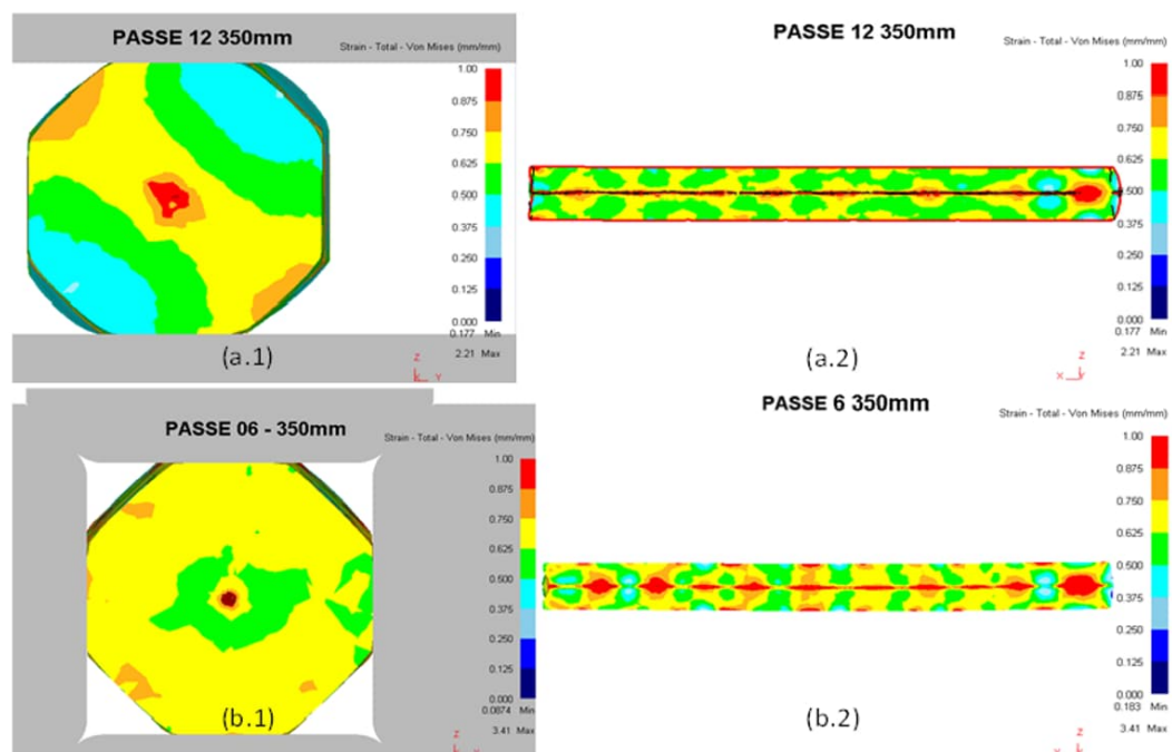
Figura 64 – Deformação de von Mises no “passe Oit 350 mm”: (a.1) 2 bigornas corte transversal e (a.2) corte longitudinal, deformações elevadas na região do vazio (cores vermelho e laranja); (b.1) 4DFD corte transversal e (b.2) corte longitudinal, deformações na região do vazio entre elevados (cores vermelho e laranja), intermediários (cores verde e amarelo) e baixos (cores azul turquesa e azul claro).
