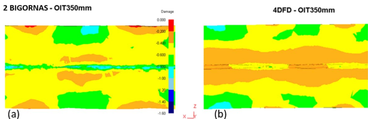
Figura 68 – Parâmetro Q -valor no “passe Oit 350 mm”: (a) 2 bigornas, valor igual a 0,8 \pm 0,2 (cores verde e azul turquesa); (b) 4DFD, valor igual a 0,4 \pm 0,2 (cores laranja e amarelo).
