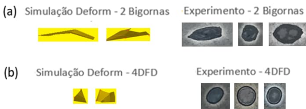
Figura 89 – Comparação das formas obtidas dos vazios nos modelos numérico (Simulação Deform) e experimental (Experimento) no oitavado de 250 mm: (a) 2 bigornas, formatos achatados no modelo numérico e alternâncias entre achatado, arredondado e ovalizado no modelo experimental; (b) 4DFD, formatos triangulares e retangulares no modelo numérico e arredondados para o experimento.
