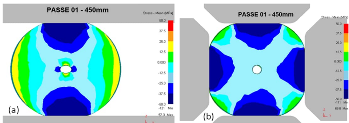
Figura 54 – Tensão hidrostática no “passe 1”: (a) 2 bigornas, tensões de tração (valores positivos nas cores amarelo e verde) e de compressão (valores negativos nas cores azul e azul escuro); (b) 4DFD, tensões de compressão (valores negativos na cor azul turquesa).
