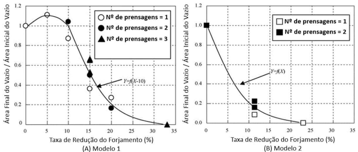
Figura 29 – Relação entre as taxas de redução e da área do vazio. Adaptado de [23].
