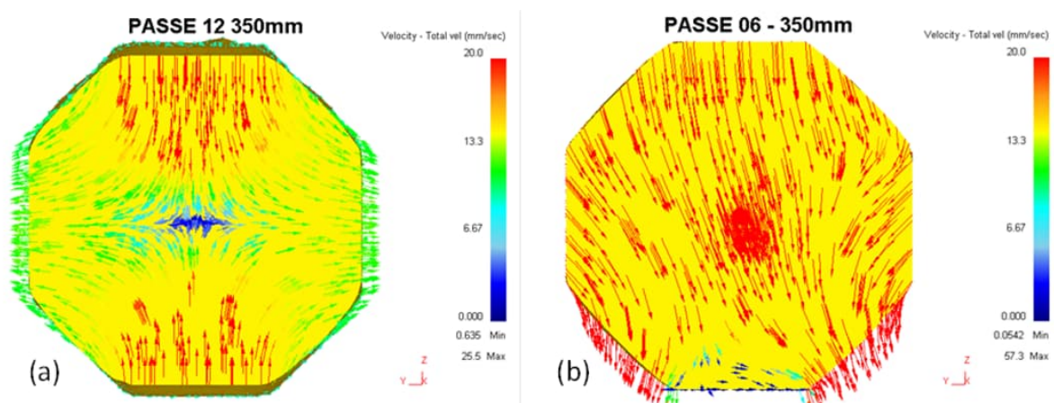
Figura 67 – Fluxo do material no “passe Oit 350 mm”: (a) 2 bigornas, fluxo inicia-se na direção Z e depois segue para as laterais na direção Y; (b) 4DFD, fluxo condicionado para o interior da barra.
