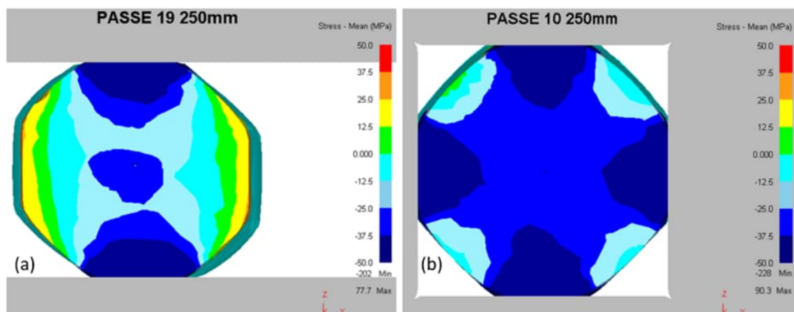
Figura 74 – Tensão hidrostática no “passage Oit 250 mm”: (a) 2 bigornas; (b) 4DFD; tensões de compressão similares (cor azul) nos dois processos ao redor do vazio.
