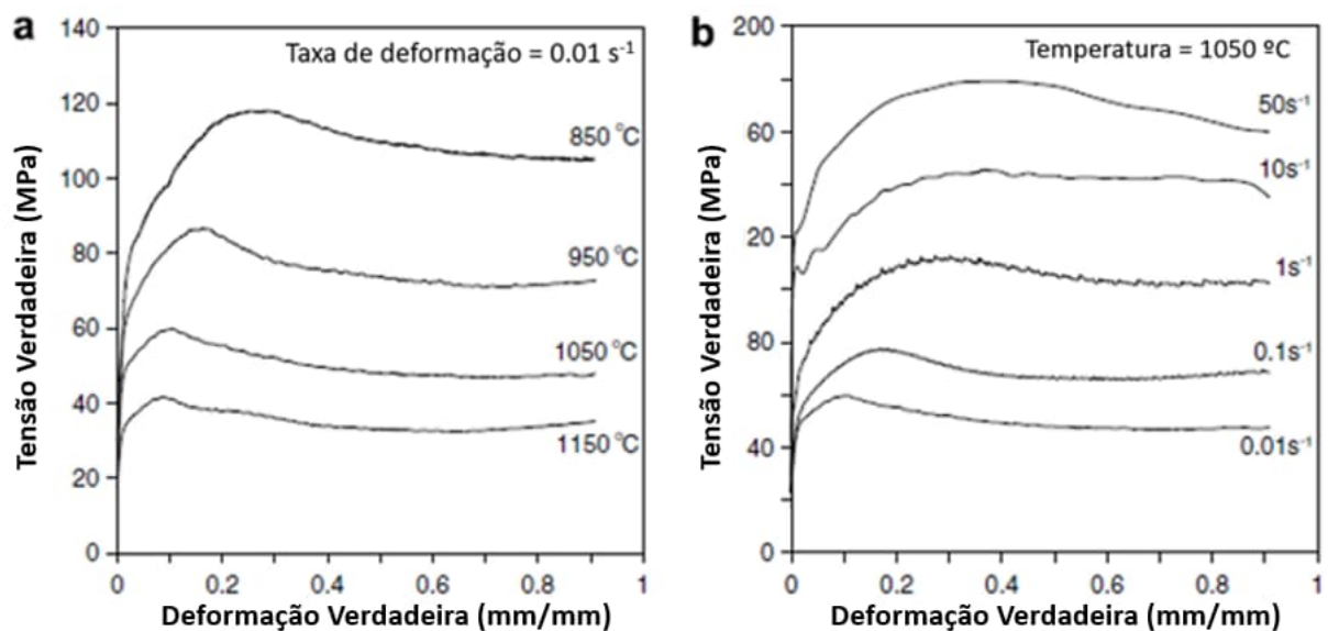
Figura 12 – Curvas típicas de tensão-deformação verdadeira para aço 42CrMo sob: (a) diferentes temperaturas de deformação; (b) diferentes taxas de deformação. Adaptado de [4].
