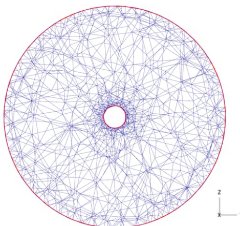
Figura 51 – Modelagem obtida pelo DEFORM TM -3D [26] com a malha da furação inicial, com 50 mm de diâmetro interno passante e 500 mm de diâmetro externo.
