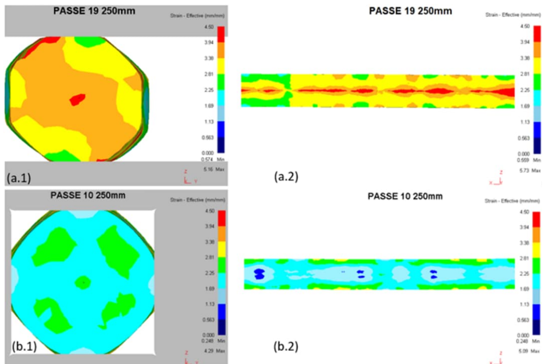
Figura 75 – Deformação efetiva no “passo Oit 250 mm”: (a.1) 2 bigornas corte transversal e (a.2) corte longitudinal; (b.1) 4DFD corte transversal e (b.2) corte longitudinal; forjamento convencional com 2 bigornas apresentou deformação efetiva maior que o forjamento com o dispositivo 4DFD.
