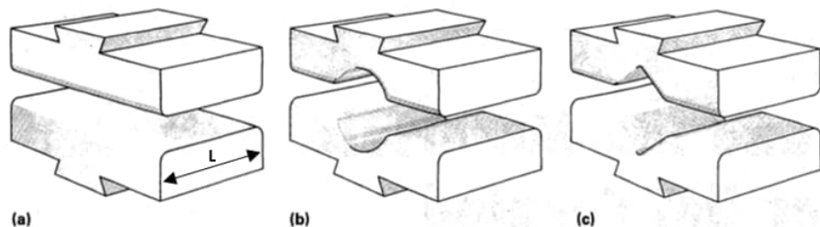
Figura 16 - Geometria de bigornas para prensas de matrizes abertas: (a) plana, onde “L” é a largura da bigorna; (b) semicircular; (c) em formato “V”. [11]
