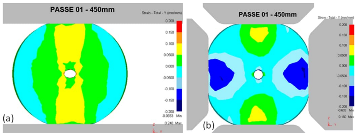
Figura 57 – Deformação total direcional Y no “passo 1”: (a) 2 bigornas, somente deformações positivas (cores verde e amarelo) em torno do vazio; (b) 4DFD, maior presença das deformações negativas (cor azul turquesa) em torno do vazio e pequena resultante de deformações positivas (cor verde).
