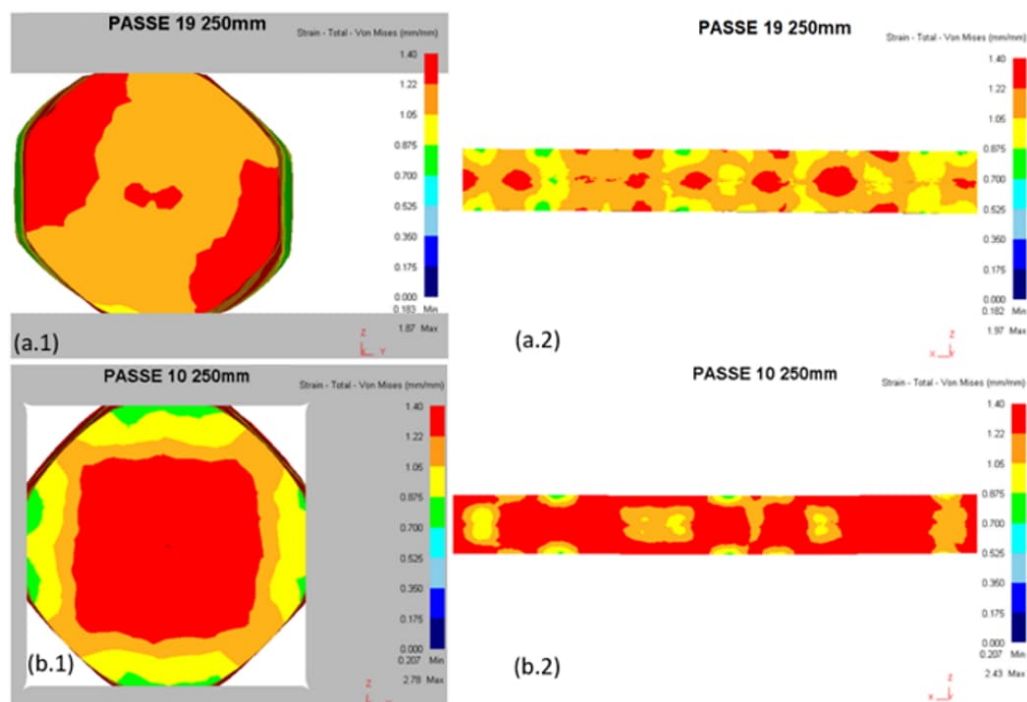
Figura 77 – Deformação de von Mises no “passe Oit 250 mm”: (a.1) 2 bigornas corte transversal e (a.2) corte longitudinal; (b.1) 4DFD corte transversal e (b.2) corte longitudinal; nos cortes transversal e longitudinal na região do vazio as deformações de von Mises foram elevadas (cores vermelha, laranja e amarelo) para os dois processos.
