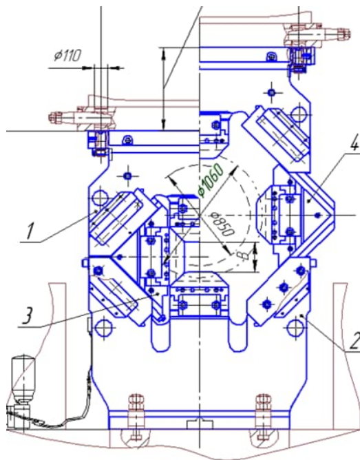
Figura 18 – Componentes principais do 4DFD: posição fechada para o alojamento superior (1) e placa corrediça (3); e posição aberta para o alojamento inferior (2) e placa corrediça (4). [13]
