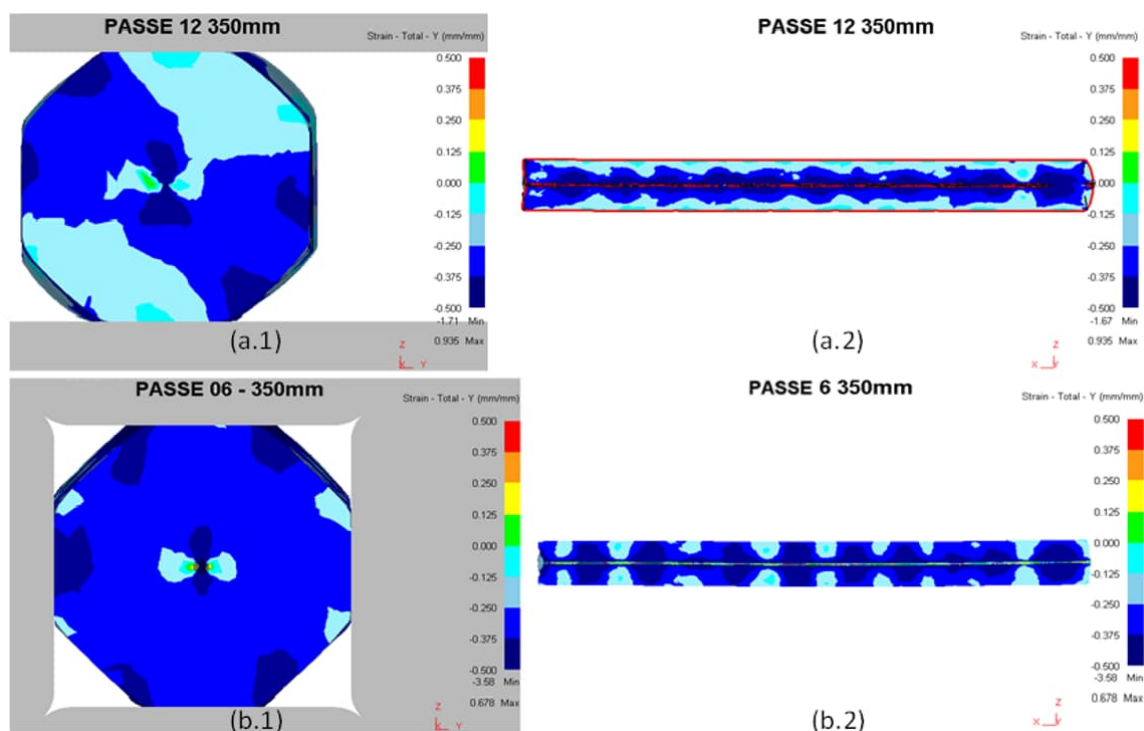
Figura 65 – Deformação total direcional Y “passo Oit 350 mm”: (a.1) 2 bigornas corte transversal e (a.2) corte longitudinal; (b.1) 4DFD corte transversal e (b.2) corte longitudinal; deformações compressivas negativas (cores azul escuro e azul claro) e uma pequena deformação trativa (cor amarela) foram semelhantes na região em torno do vazio para os dois processos.
