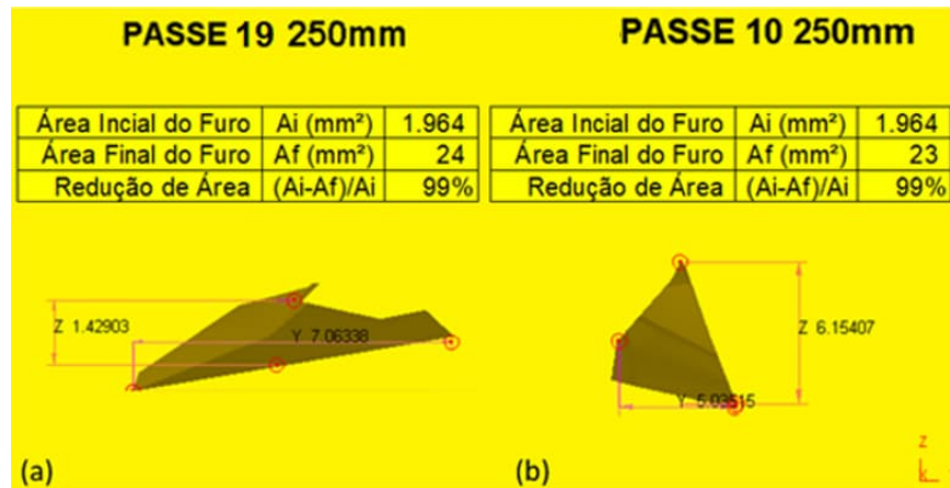
Figura 73 – Dimensão do vazio (furo) “passage Oit 250 mm”: (a) 2 bigornas, redução de área do vazio igual a 99%; (b) 4DFD, redução de área do vazio igual a 99%.
