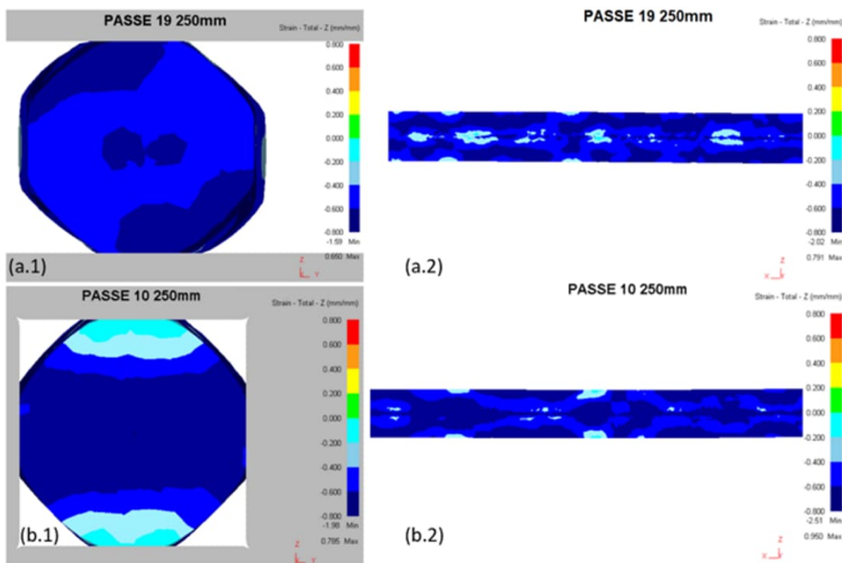
Figura 79 – Deformação total direcional Z “passe Oit 250 mm”: (a.1) 2 bigornas corte transversal e (a.2) corte longitudinal; (b.1) 4DFD corte transversal e (b.2) corte longitudinal; deformação compressiva maior (cor azul escuro) para o 4DFD e alternância de níveis das deformações compressivas (cores azul, azul escuro e azul claro) no processo com 2 bigornas ao longo da região central do vazio.
