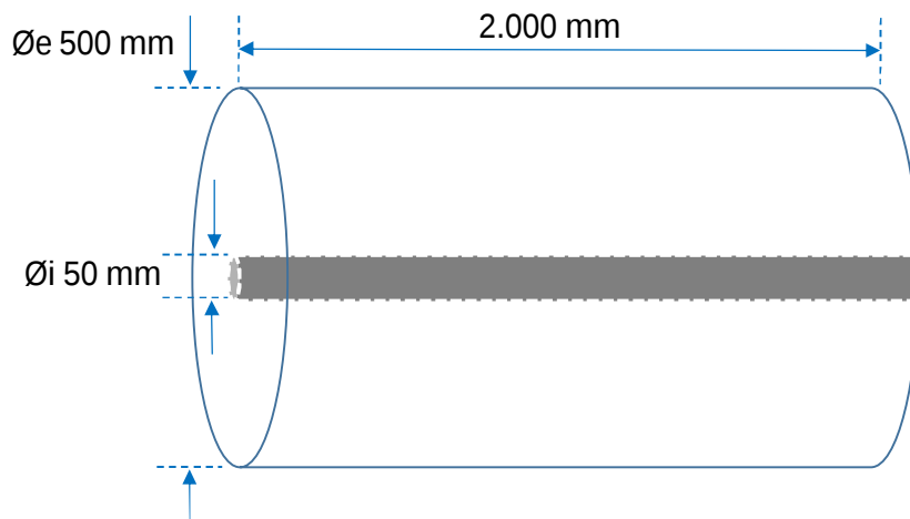
Figura 41 – Representação esquemática da geometria inicial das barras.
