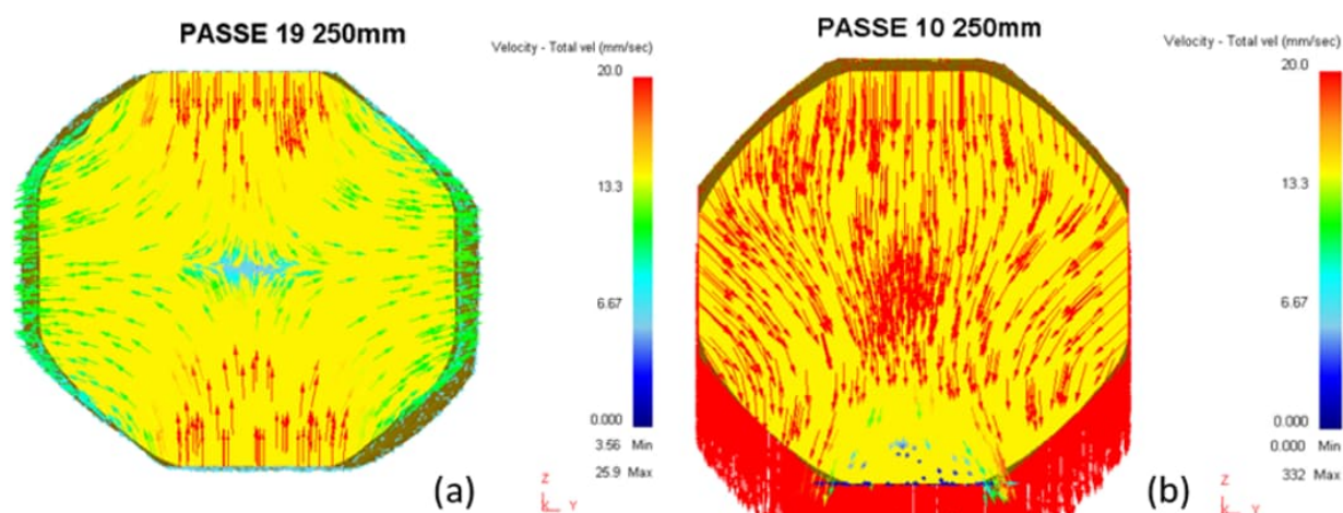
Figura 80 – Fluxo do material no “passe Oit 250 mm”: (a) 2 bigornas, fluxo inicia-se na direção Z e depois segue para as laterais na direção Y; (b) 4DFD, fluxo condicionado para o interior da barra.
