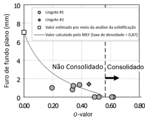
Figura 26 – Variação do tamanho do defeito em mm com o Q -valor, equação (41). Adaptado de [22].
