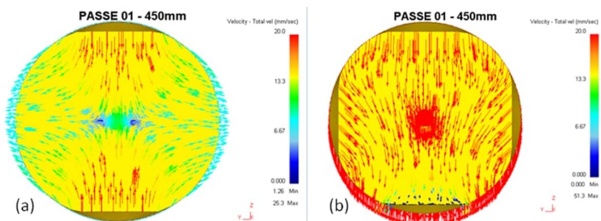
Figura 59 – Fluxo do material no “passe 1”: (a) 2 bigornas, fluxo inicia-se na direção Z e depois segue para as laterais na direção Y; (b) 4DFD, fluxo condicionado para o interior da barra.
