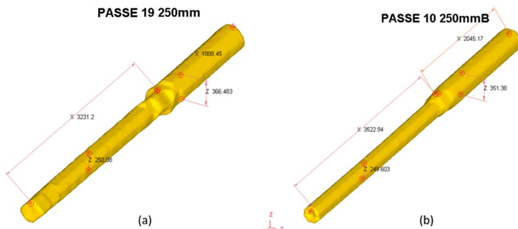
Figura 69 – Geometria 3D no “passe Oit 250 mm”: (a) 2 bigornas, 250,08 por 3.231,2 mm de comprimento; (b) 4DFD, 249,60 mm por 3.522,9 mm.
