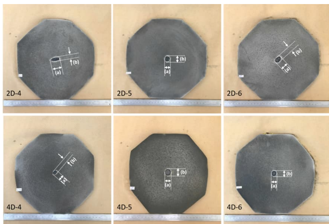
Figura 86 – Macrografias das fatias no formato oitavado 250 mm: 2 bigornas planas (2D-4, 2D-5 e 2D-6); dispositivo 4DFD (4D-4, 4D-5 e 4D-6); dimensões (a) e (b) dos vazios encontram-se na Tabela 12.
