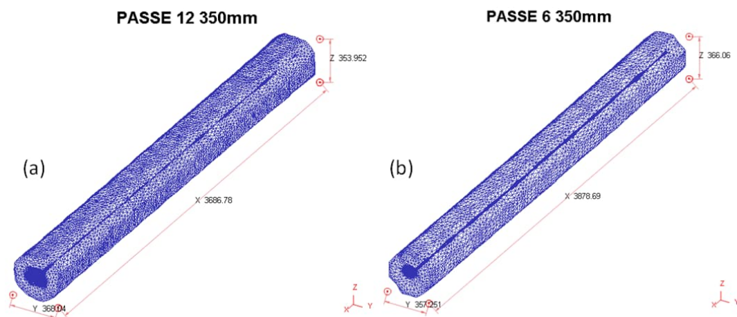
Figura 60 – Geometria 3D no “passe Oit 350 mm”: (a) 2 bigornas, 354 mm e 368 mm por 3.687 mm de comprimento; (b) 4DFD, 357 mm e 366 mm por 3.879 mm.
