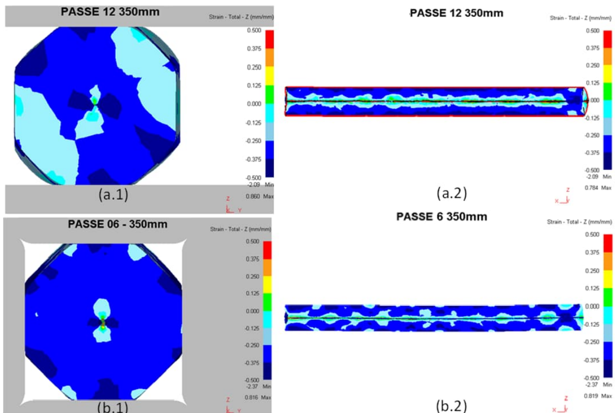
Figura 66 – Deformação total direcional Z “passe Oit 350 mm”: (a.1) 2 bigornas corte transversal e (a.2) corte longitudinal; (b.1) 4DFD corte transversal e (b.2) corte longitudinal; deformações compressivas negativas (cores azul, azul escuro e azul claro) e uma pequena deformação trativa (cor amarela) foram semelhantes na região em torno do vazio para os dois processos.
