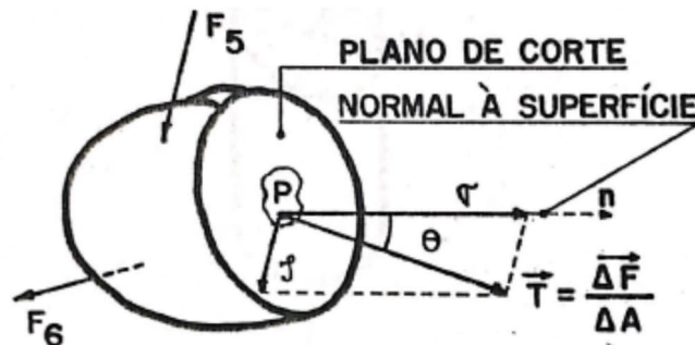
Figura 1 – Decomposição da tensão T segundo eixos cartesianos. [1]
