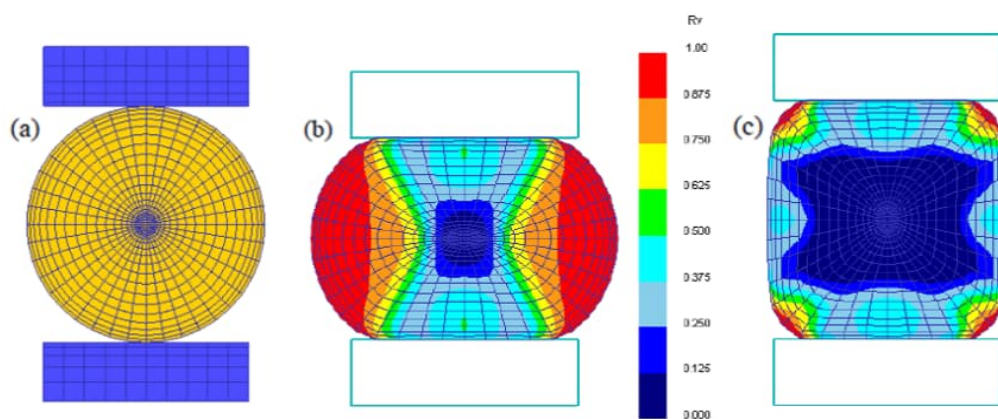
Figura 24 – Simulação por elementos finitos para o volume relativo de vazios (Rv): (a) bigorna plana; (b) Rv após redução de 24%; (c) Rv após rotação de 90^\circ de (b), seguido de redução de 22%. [19]
