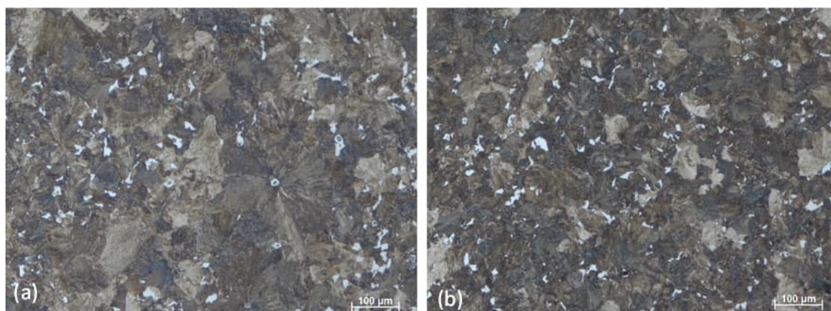
Figura 94 – Micrografias da superfície do oitavado 250 mm: (a) 2 bigornas; (b) 4DFD; microestrutura perlítica e ferrítica; tamanho de grão mais grosseiro para o processo com 2 bigornas, com 3 ASTM, do que para o 4DFD, igual a 5 ASTM. Ataque Nital 4%. Aumento 100x.
